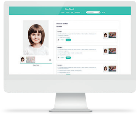
INTERFACE FAMILLE
