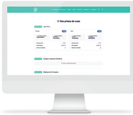
INTERFACE ÉTABLISSEMENT
